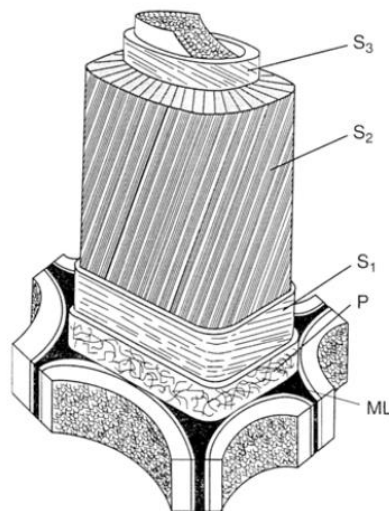
Figure 1.3 : Schéma de la structure de la paroi cellulaire secondaire avec agencement de l'angle des microfibrilles des différentes couches S (S1, S2 et S3). (Booker and Sell, 1998)
